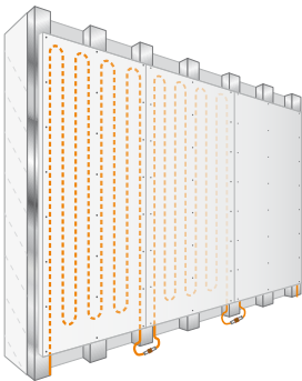
PareteModuloStandard
