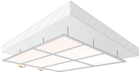
Sistema classic in reticolo soffitto
