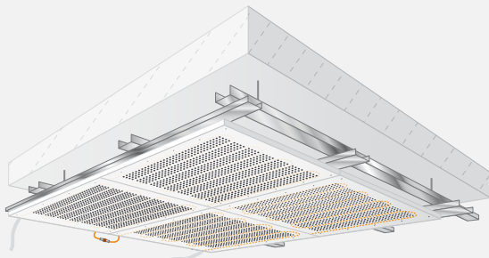
SoffittoModuloStandard Acustico
